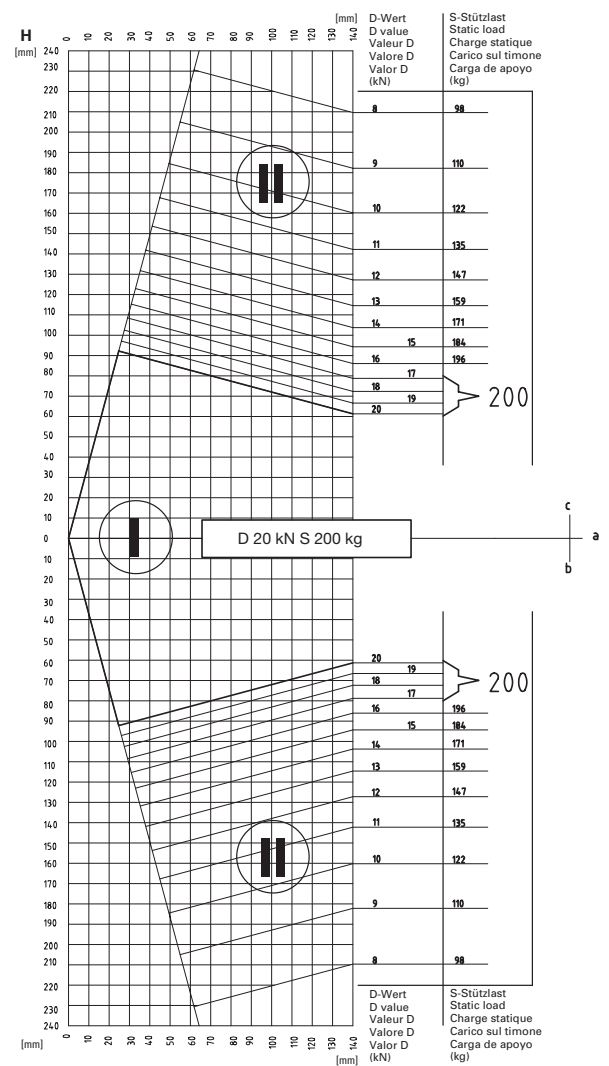
ISO 85 x 45
